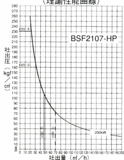
(理論性能曲線)
